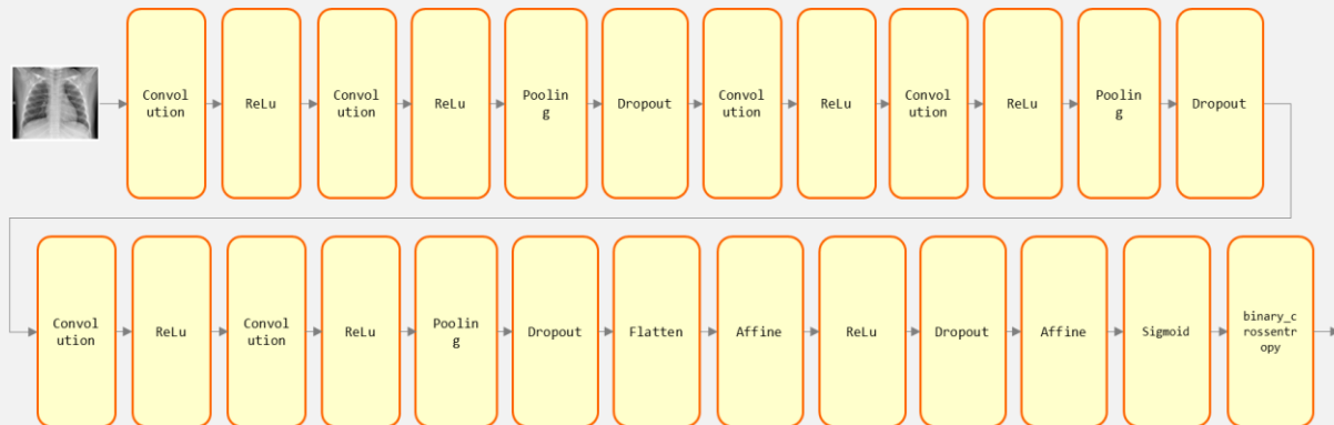
인공지능망 네트워크 구성
